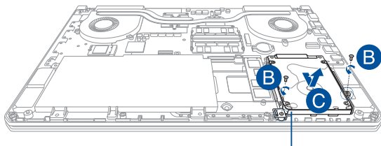
відсік для жорсткого диска
